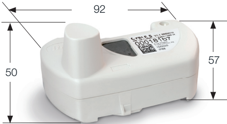
Abmessungen (mm)
